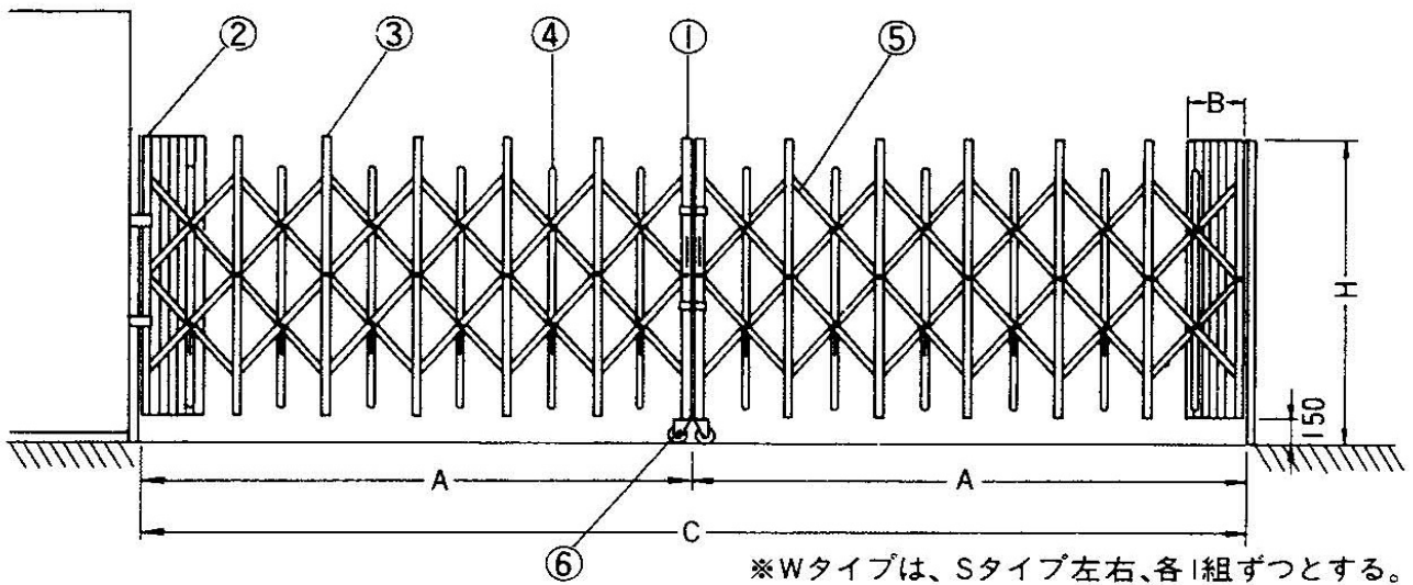
(正面図)
